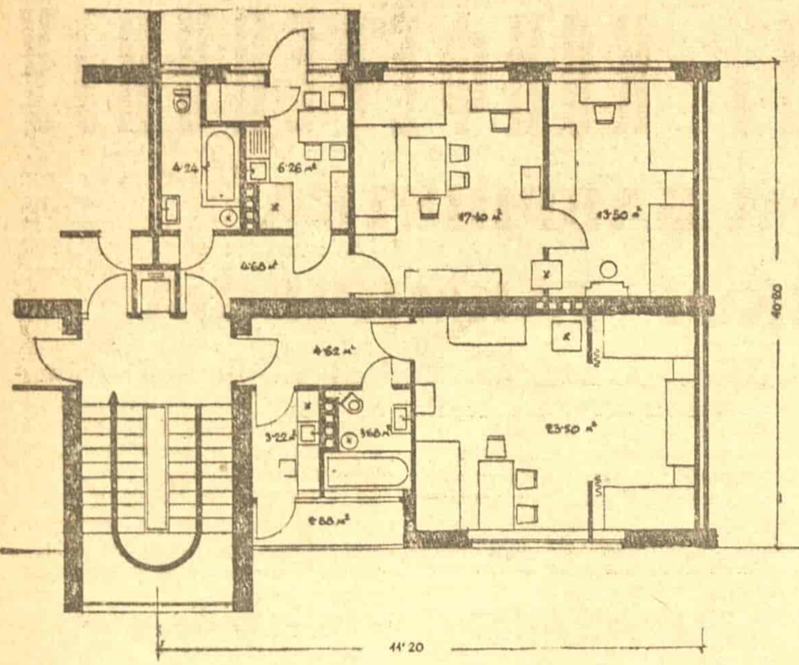
Један предлог за распоред станбеног простора
