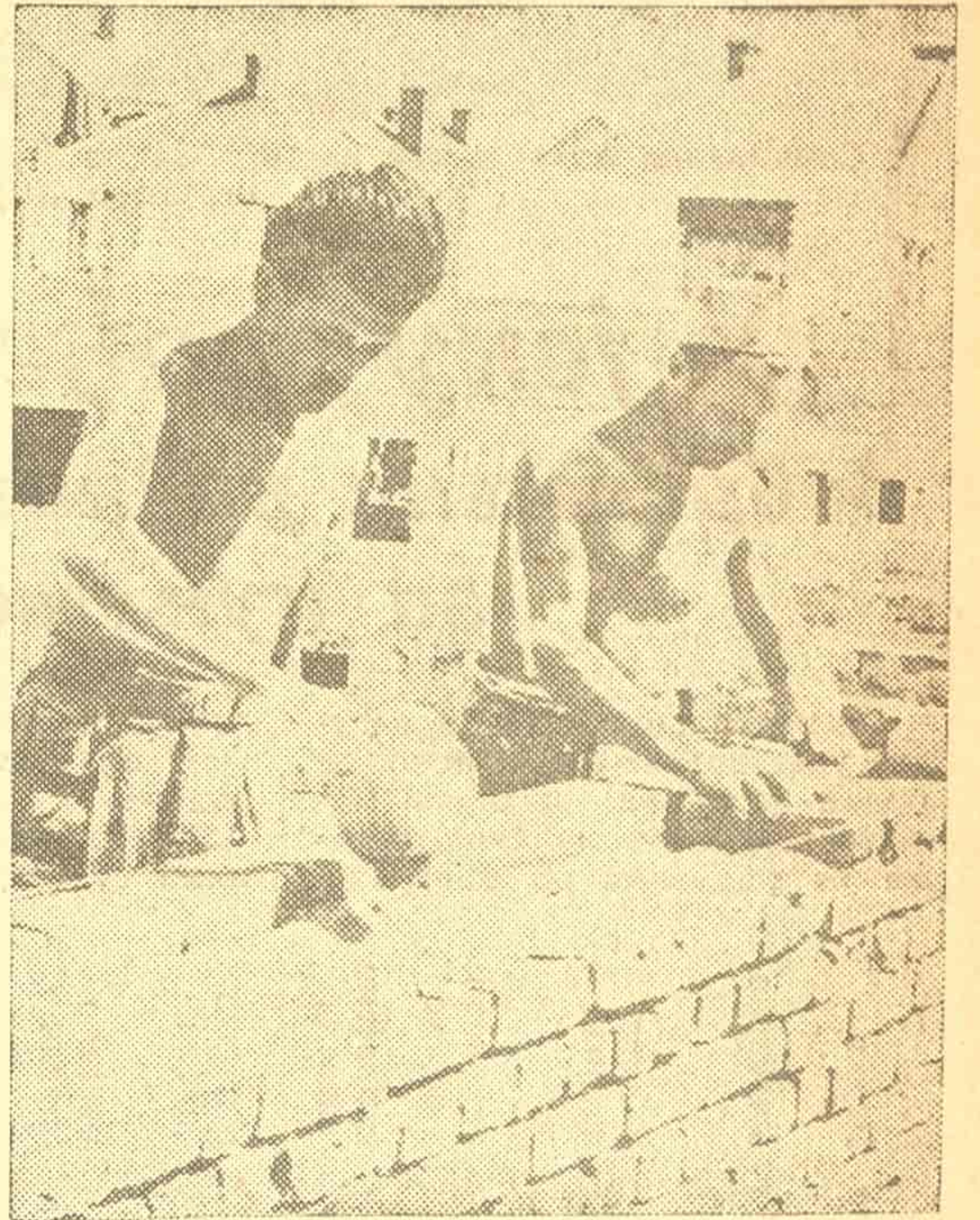
«Двојка» из бригаде Марка Марјановића која примењује нов начин зидања на станбеним зградама у Цвијичевој улици. Сви радници из бригаде Марјановића примењују нову методу рада и служе као пример осталим својим друговима.
