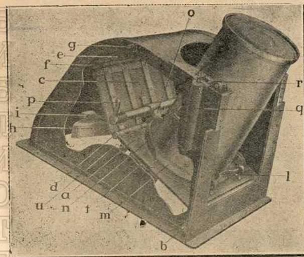
Сл. 22. — Затварач „Es—Em“ у тренутку кад се суд излучује
