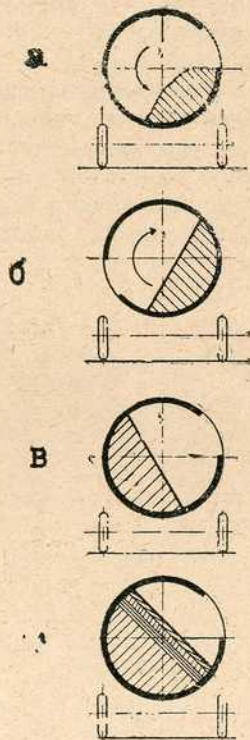
Сл. 14. — Шема пуњења сандука са затварачима
