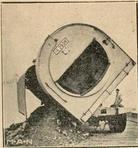
Сл. 18. — Аутомобил за сметлиште фирме М.А.Н.
