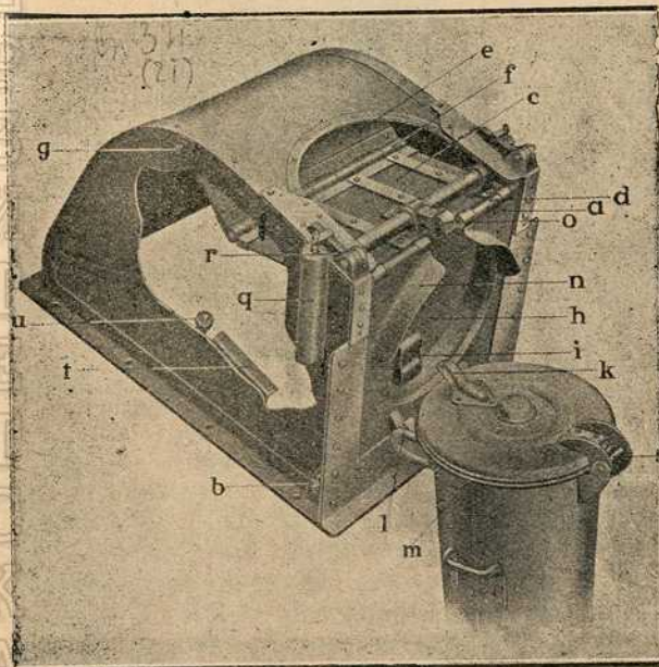
Сл. 21. — Затварач „Es—Em“ у тренутку кад се суд заклопи
