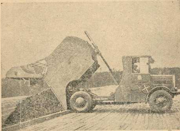
Сл. 17 а. — Изручивање сметлишта аутомоб. Гаип
