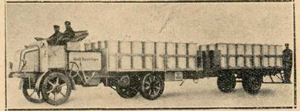
Сл. 19. — Аутомобил за систем мењања судова
