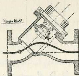
Сл. 4. — Вентил конструкције „Косва”.
