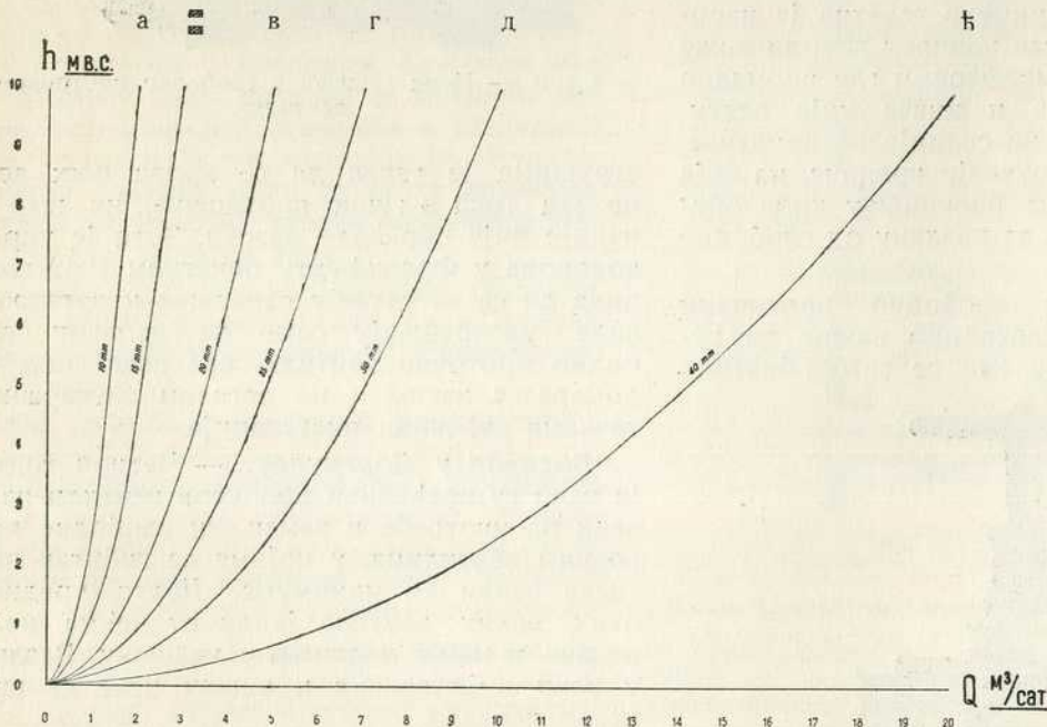
Графикон губитка притиска у водомерима типа Бол и Ројтер, за калибре до 40 мм. закључно.
