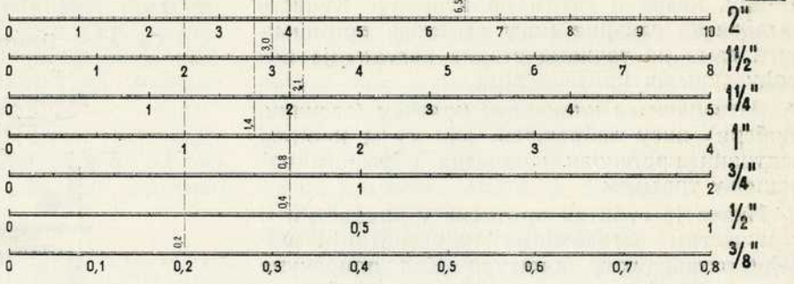
Графикон губитка притиска у затварачким вентилима, односно у течећим славинама, у зависности од протицајне количине воде. — Састављено по испитивањима инжењера Г. Физона, 33 калибре од \frac{3}{8} " до 2".
