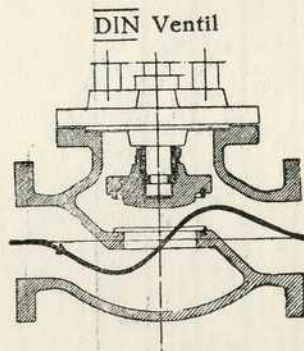
Сл. 3. — Нормални вентил ДИН.
