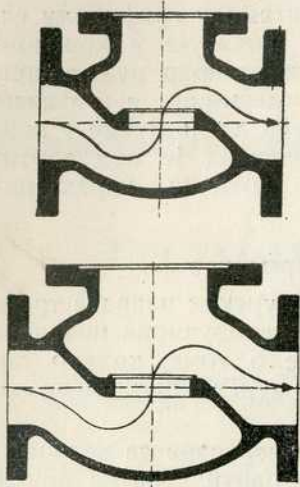
Сл. 6. — Кутија обичног досад затварачког вентила.
