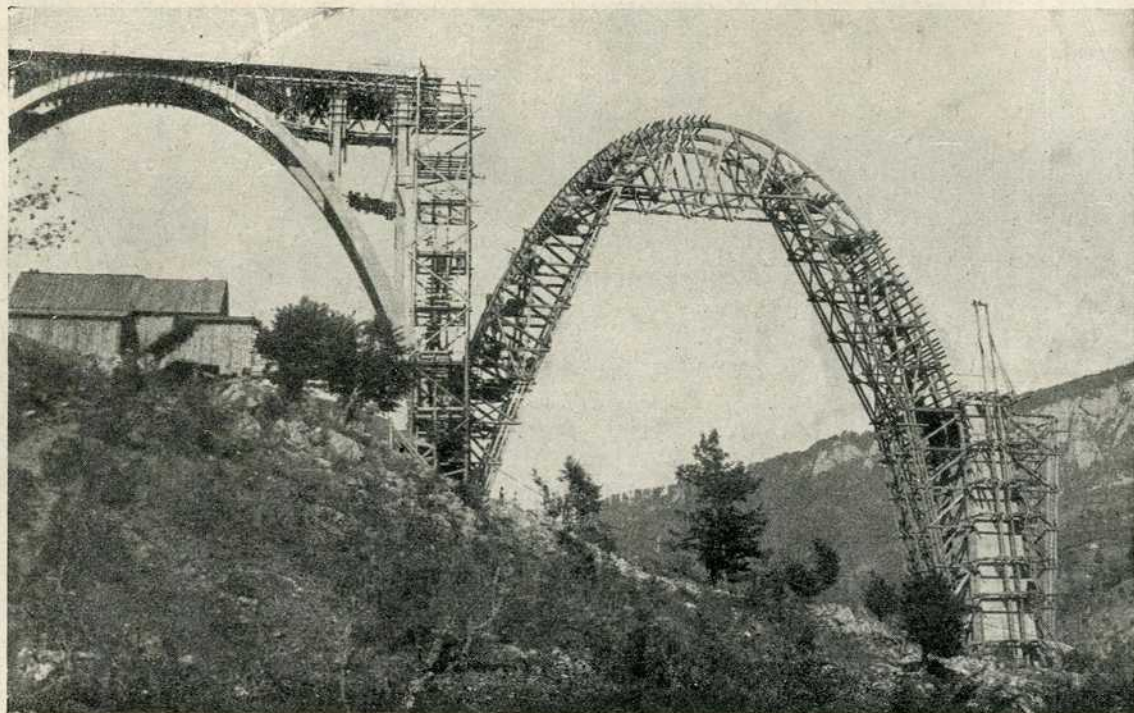
Мост на Тари у изградњи
