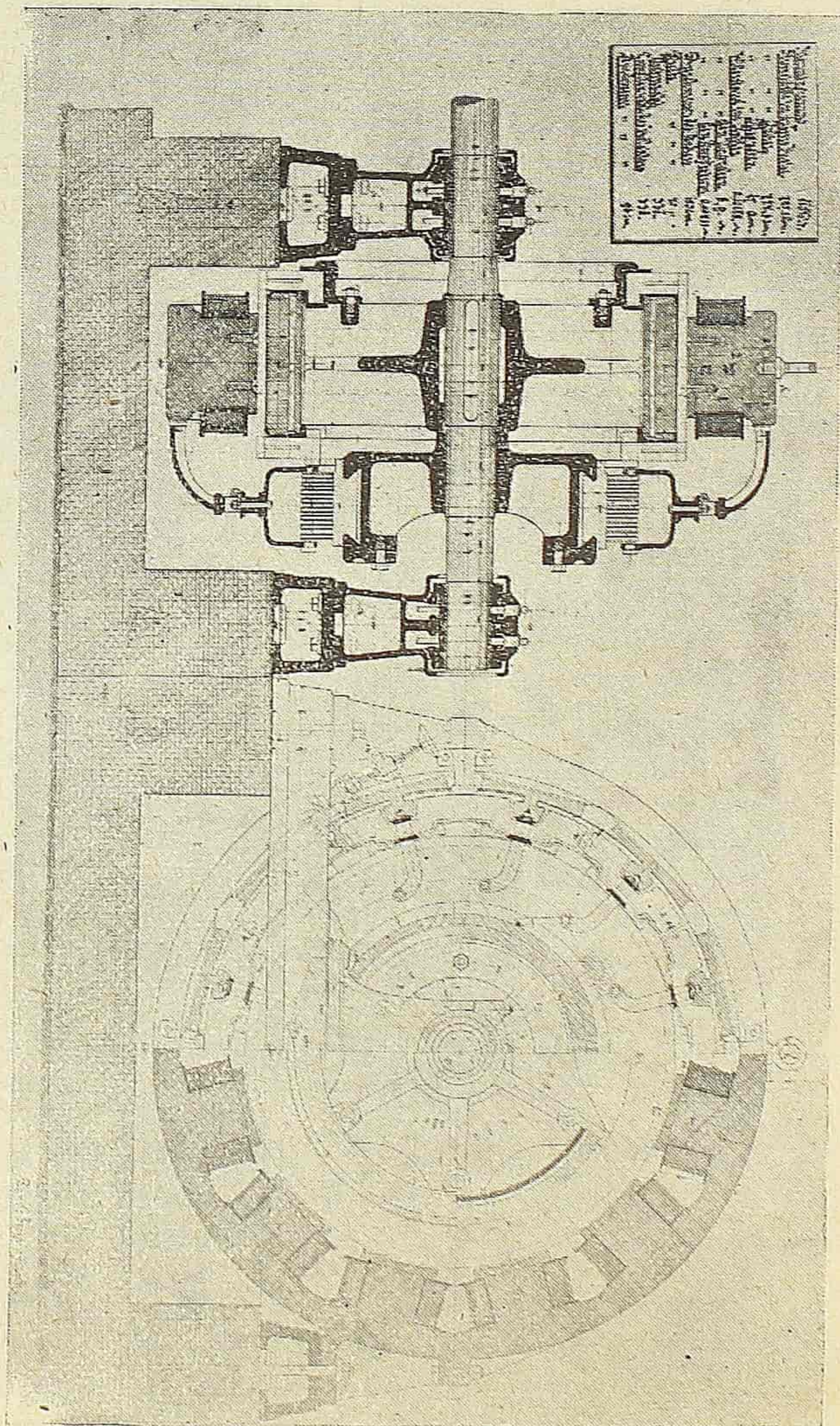
Пројект-план динамо-машине за електрично осветљење.
