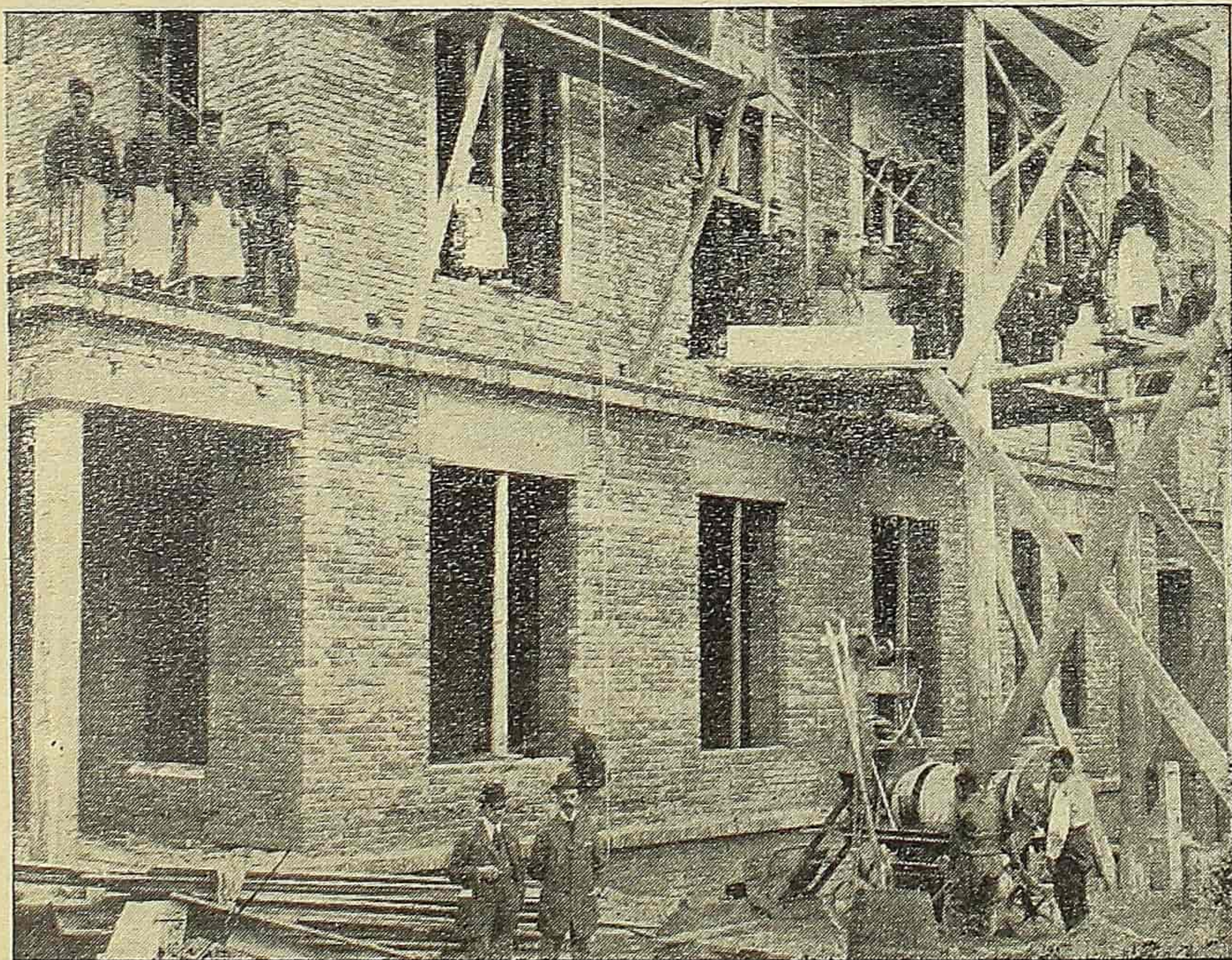
Санаторијум — Врачар (при зидању).
